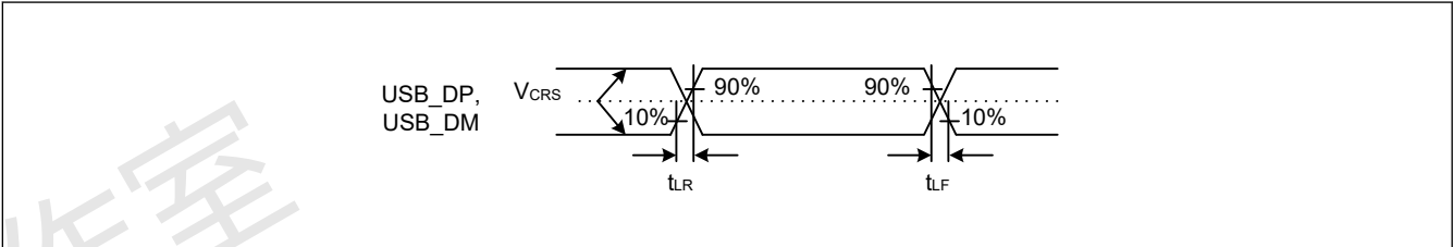
Figure 2.54 低速模式下的USB_DP和USB_DM输出时序
