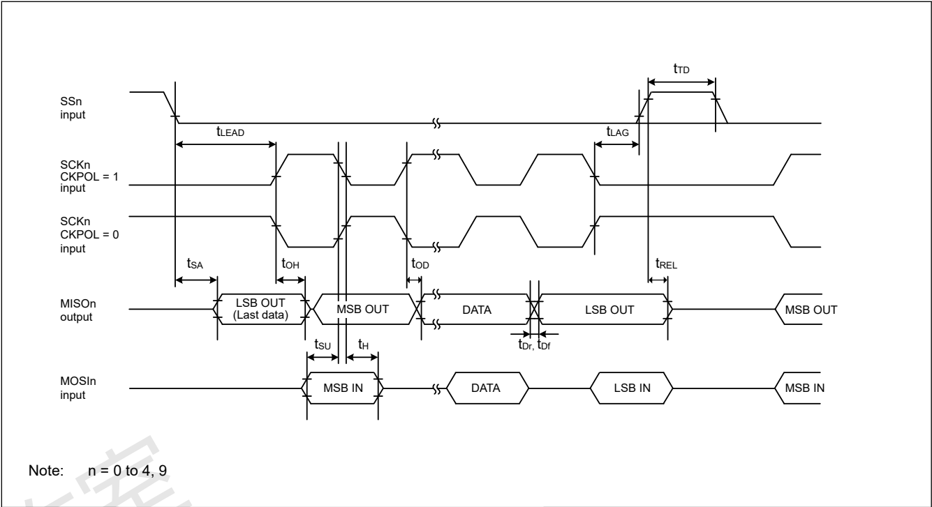
Figure 2.31 CKPH=0时从机的SCI简单SPI模式时序
