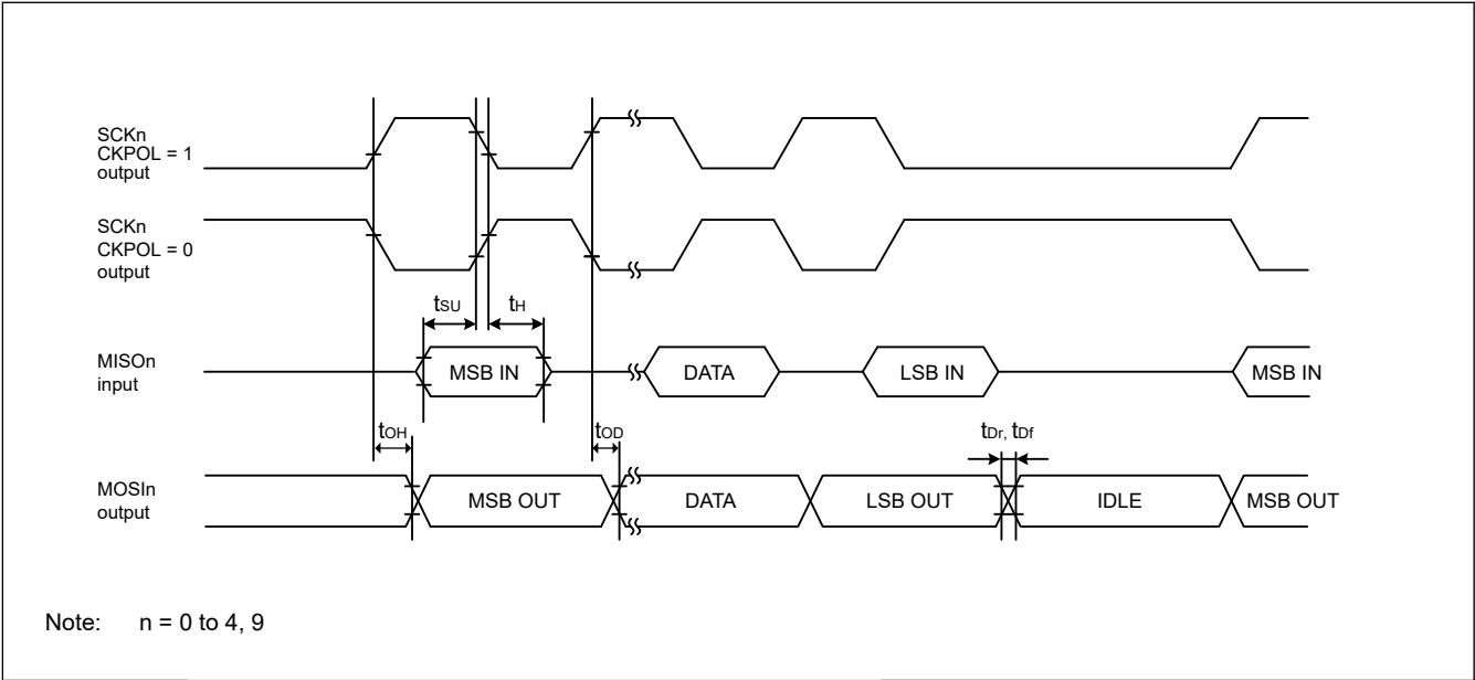
Figure 2.29 CKPH=0时主机的SCI简单SPI模式时序
