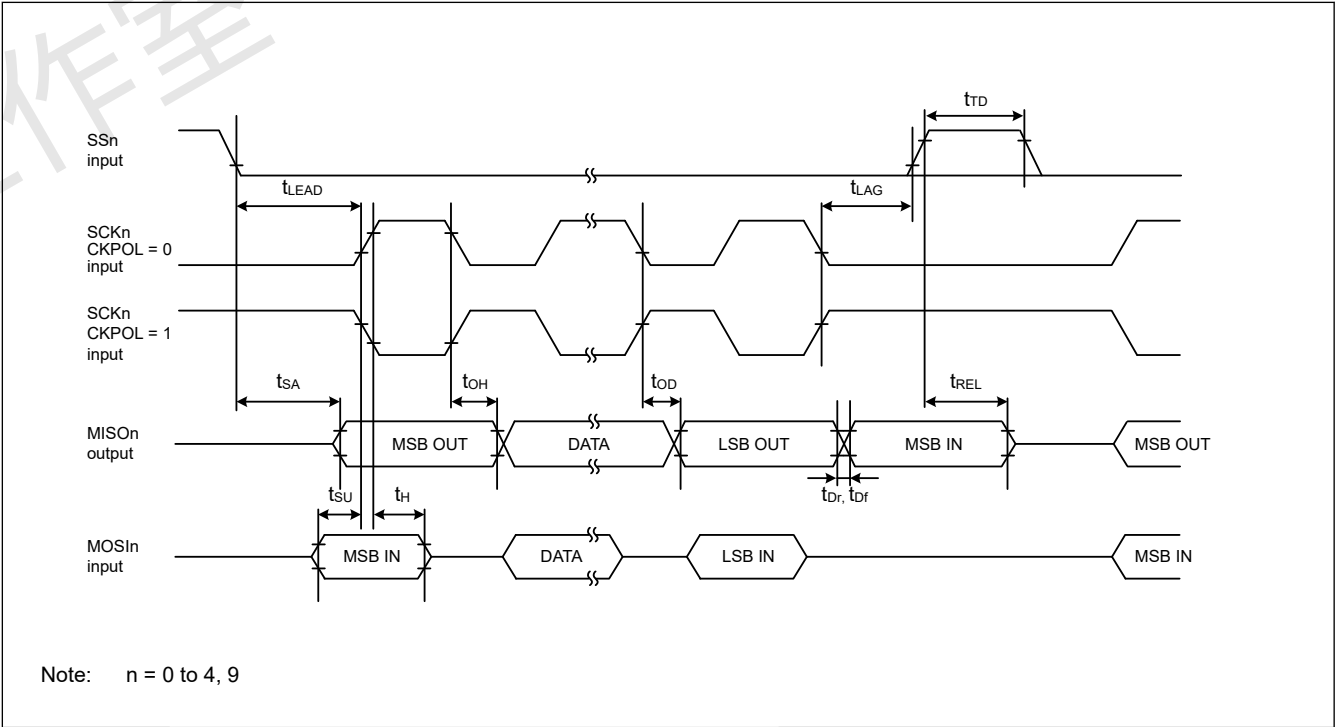
Figure 2.30 CKPH=1时从机的SCI简单SPI模式时序
