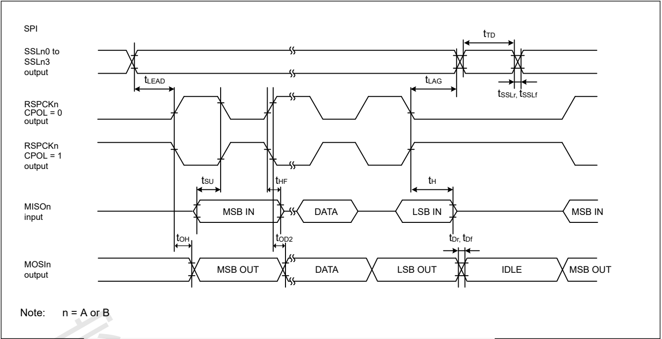
Figure 2.37 当CPHA=1且比特率设置为PCLKA/2时, 主机的RSPI时序
