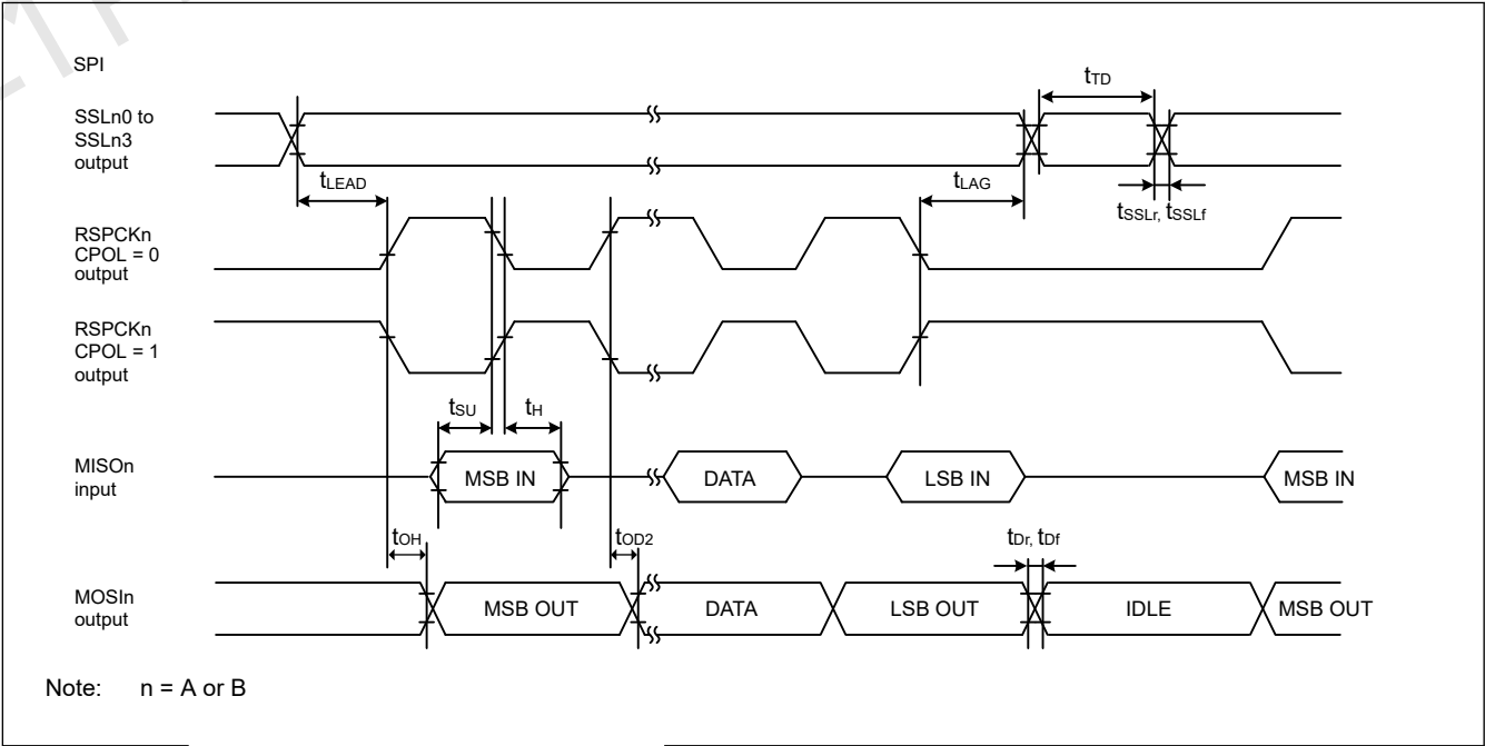
Figure 2.36 CPHA=1时主机的SPI时序
