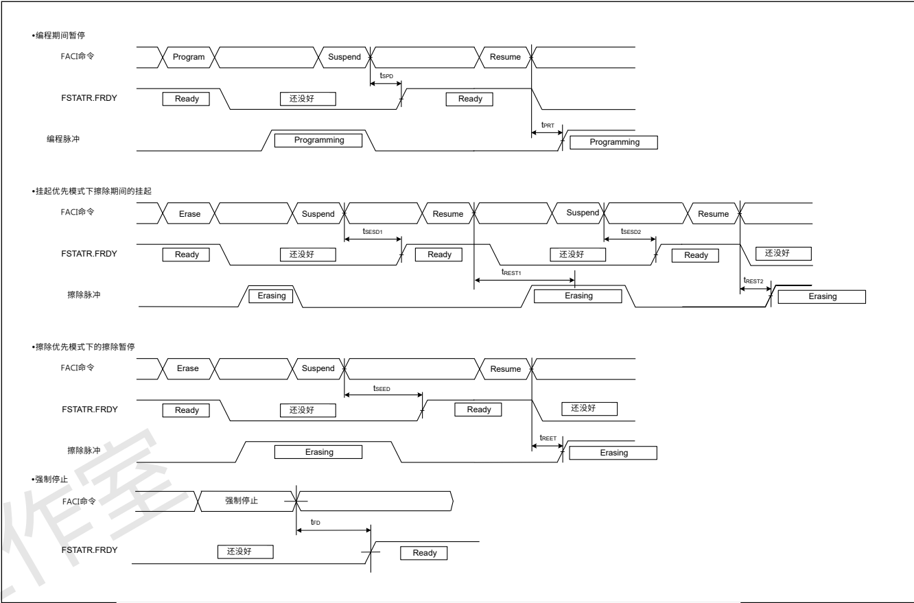
Figure 2.66 闪存编程和擦除的暂停和强制停止时序
