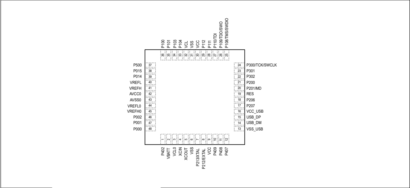
Figure 1.5 QFN48引脚的引脚分配
