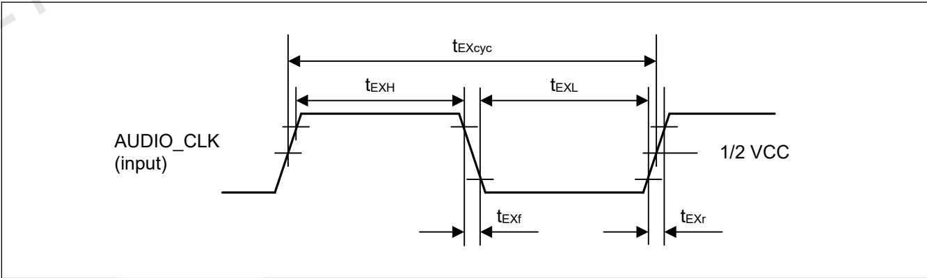
Figure 2.44 时钟输入时序
