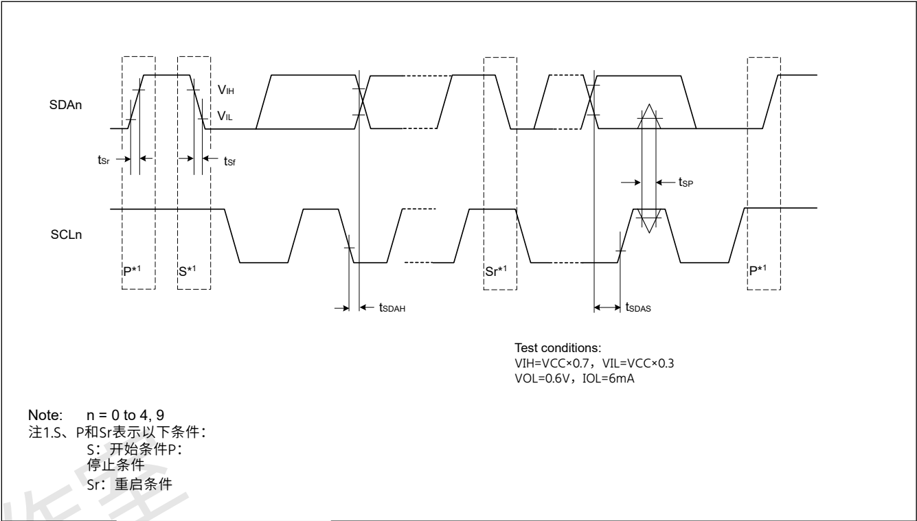
Figure 2.32 SCI简单IIC模式时序
