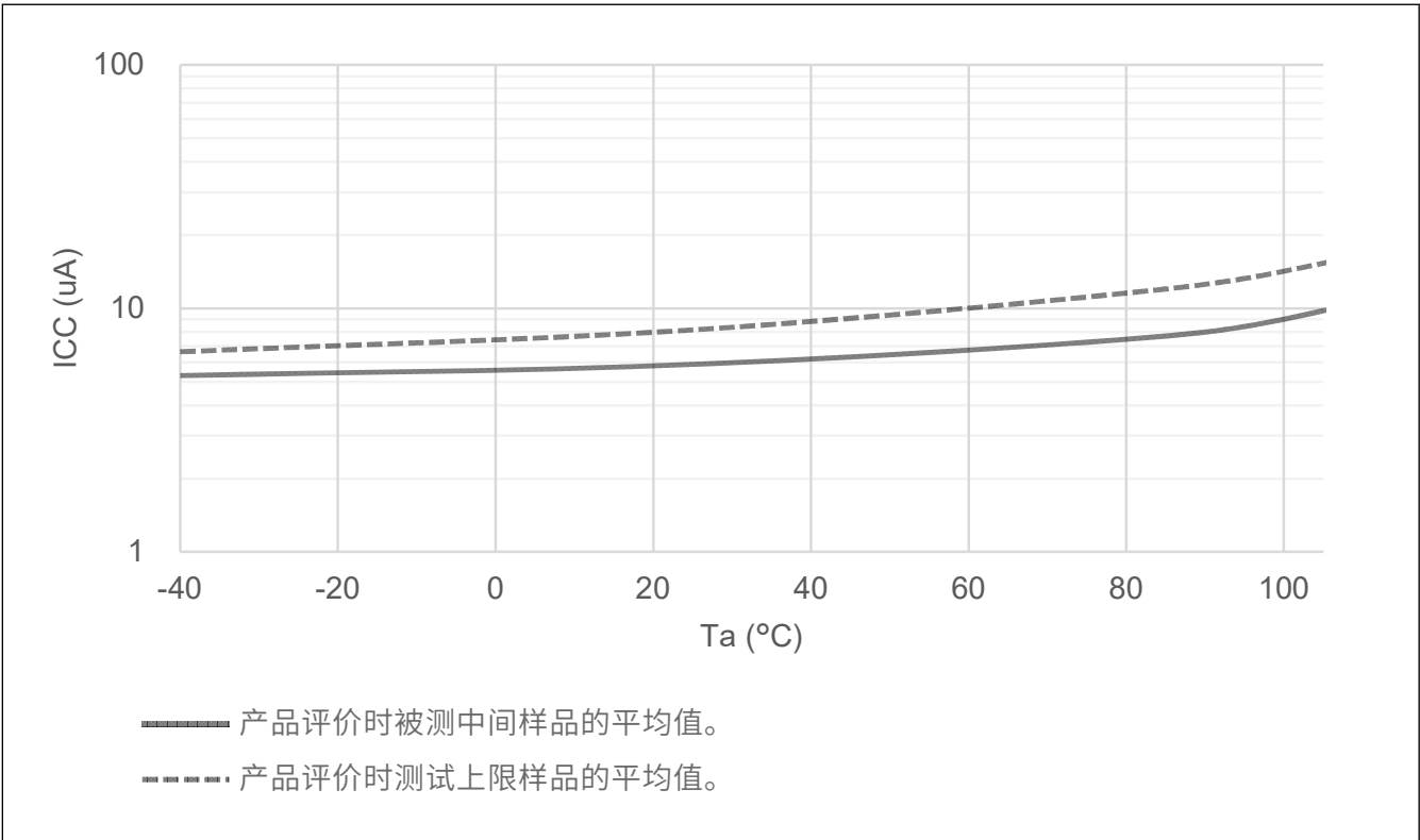
Figure 2.5 深度软件待机模式下的温度依赖性，未向SRAM供电或USB恢复检测单元，上电复位电路低功耗功能启用（参考数据）
