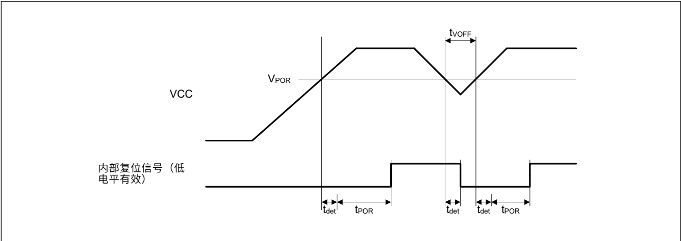
Figure 2.60 上电复位时序
