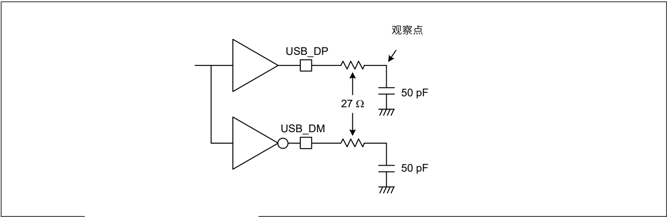
Figure 2.57 全速模式下的测试电路
