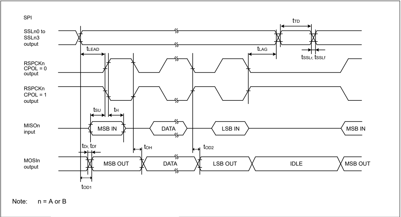
Figure 2.34 CPHA=0时主机的SPI时序
