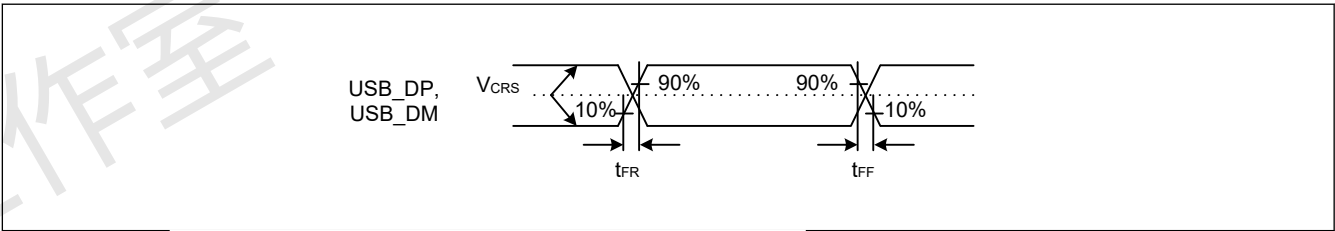
Figure 2.56 全速模式下的USB_DP和USB_DM输出时序
