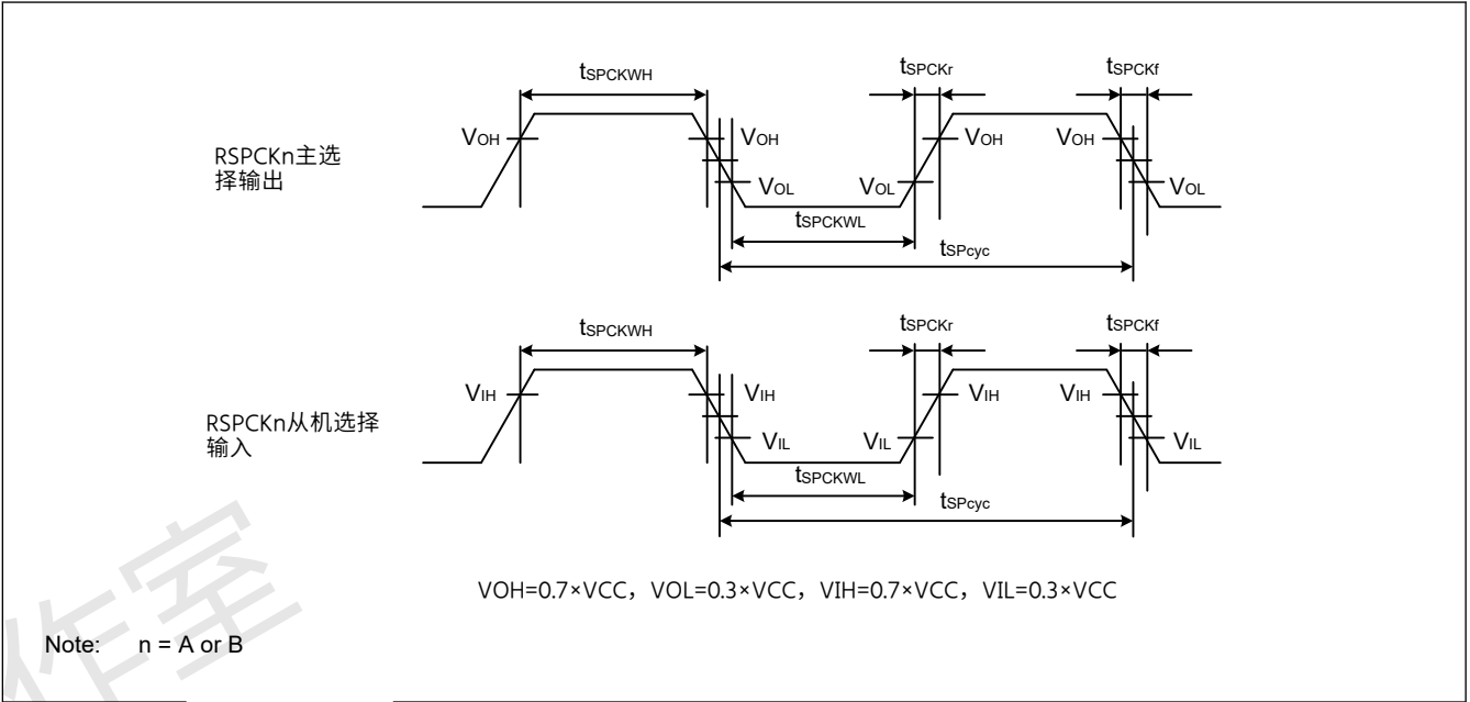
Figure 2.33 SPI时钟时序
