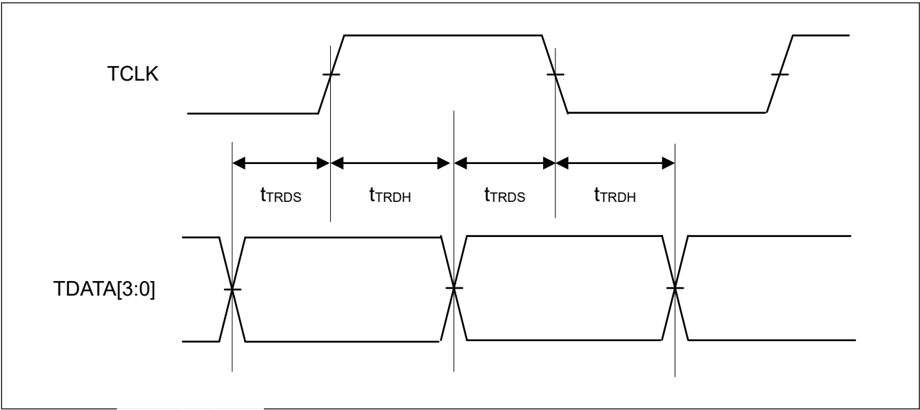
Figure 2.75 ETM输出时序
