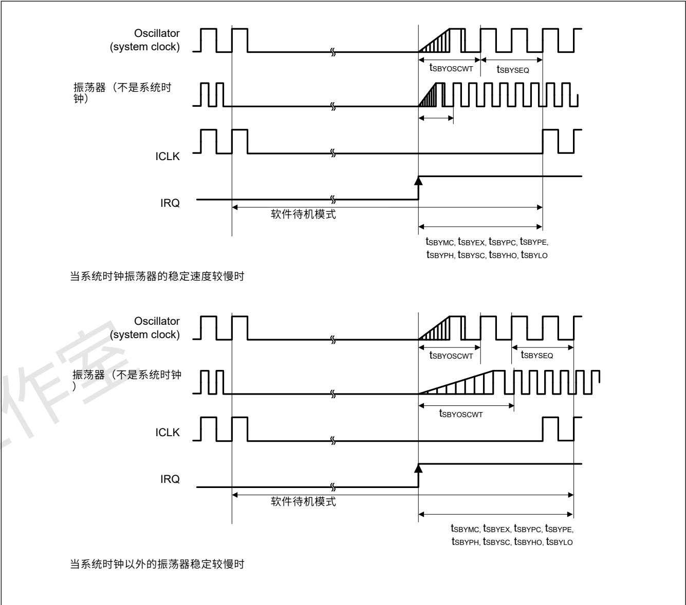
Figure 2.14 软件待机模式取消时序
