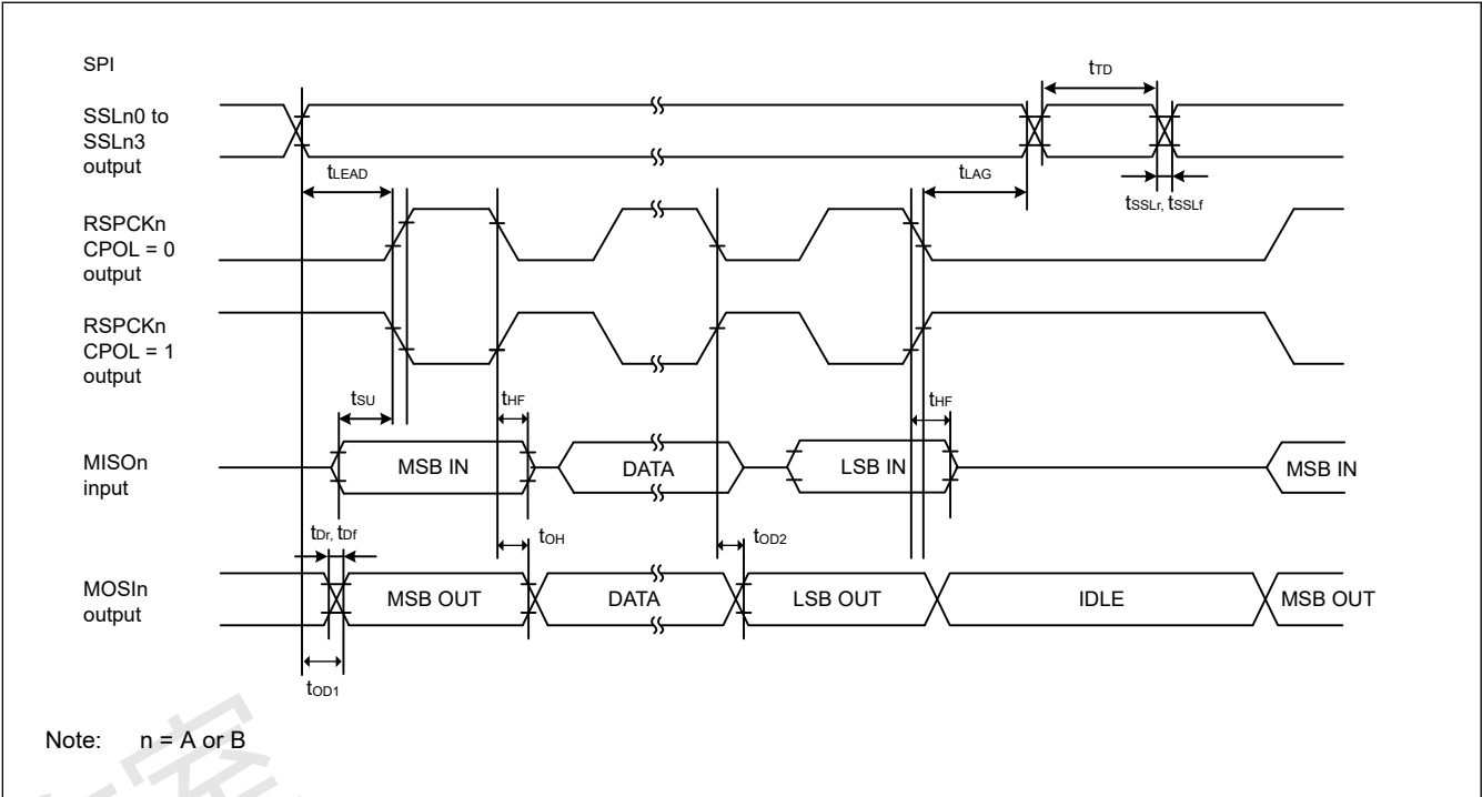
Figure 2.35 当CPHA=0且比特率设置为PCLKA/2时主设备的SPI时序
