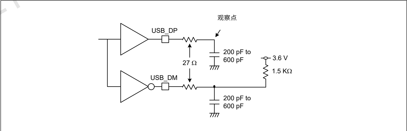
Figure 2.55 低速模式下的测试电路
