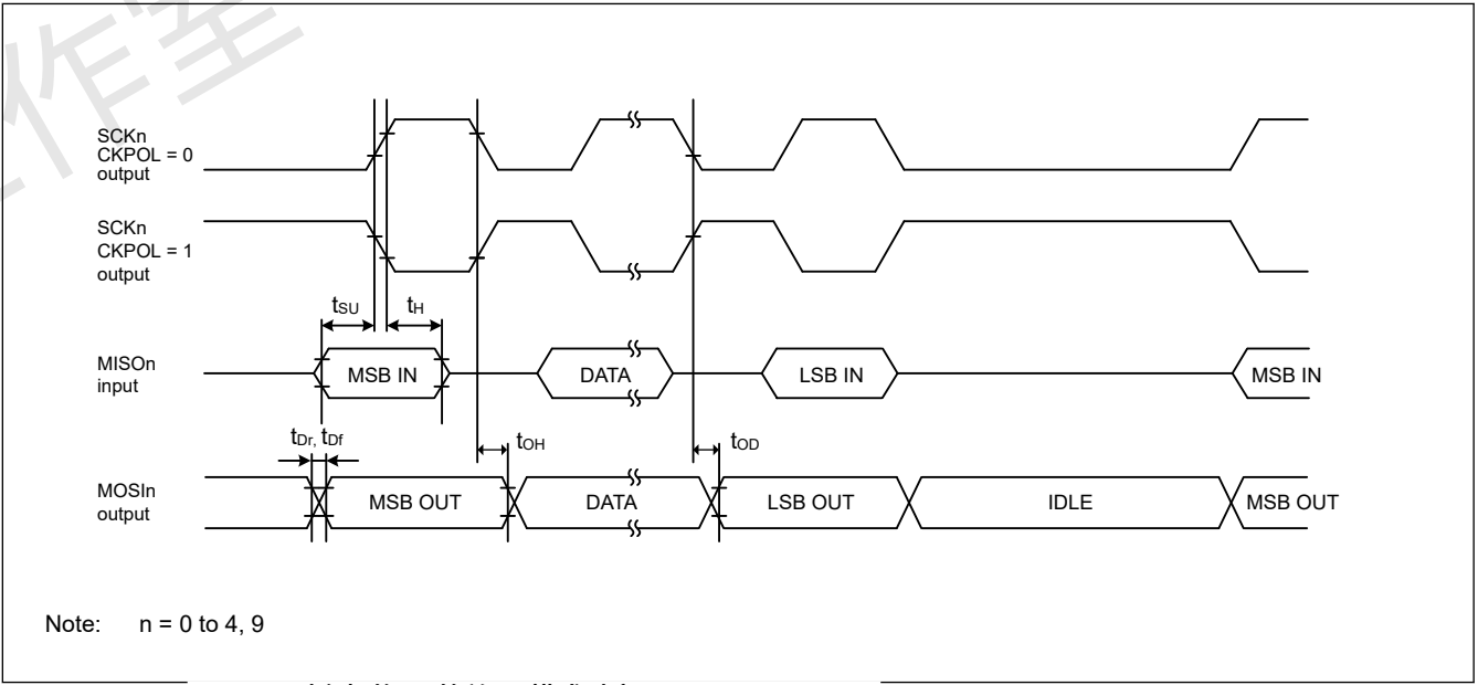
Figure 2.28 CKPH=1时主机的SCI简单SPI模式时序
