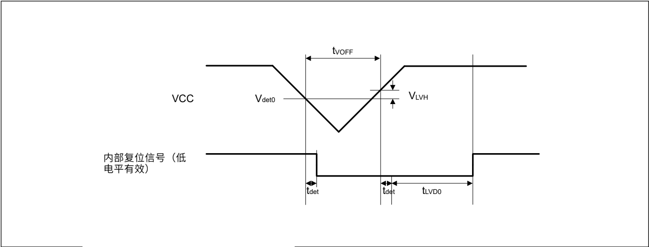
Figure 2.61 电压检测电路时序 (V det0 )
