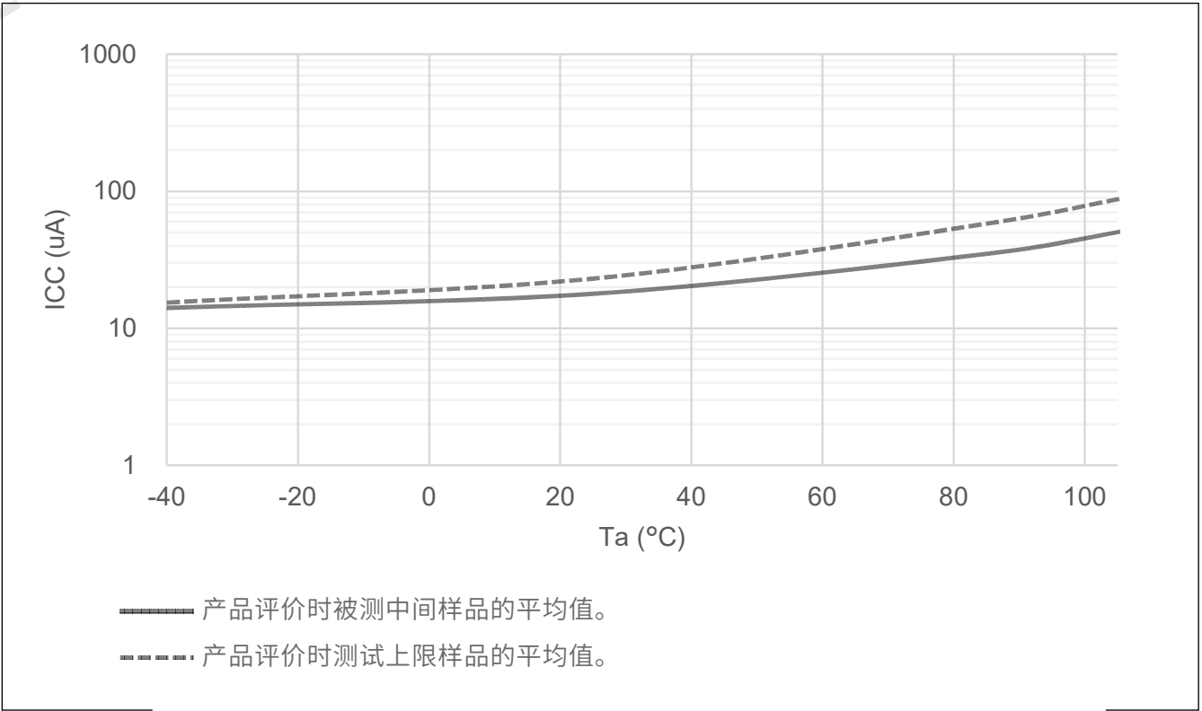
Figure 2.3 深度软件待机模式下的温度依赖性、为待机SRAM和USB恢复检测单元供电（参考数据）
