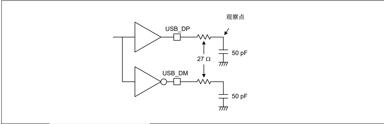
Figure 2.53 全速模式下的测试电路
