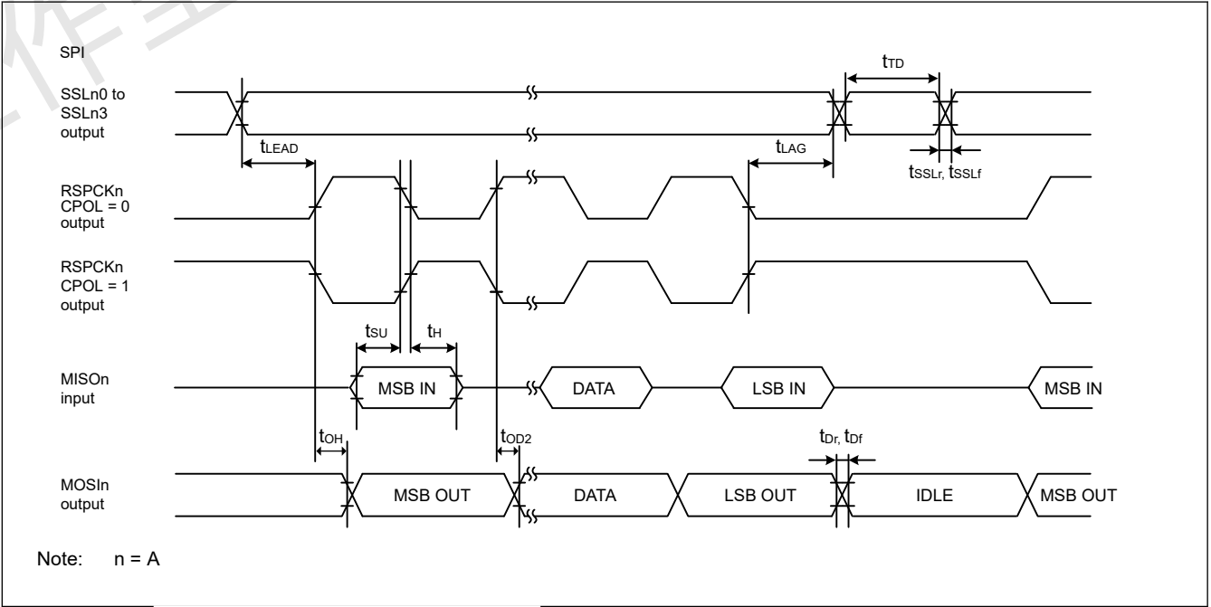
Figure 2.37 CPHA=1时主设备的SPI时序
