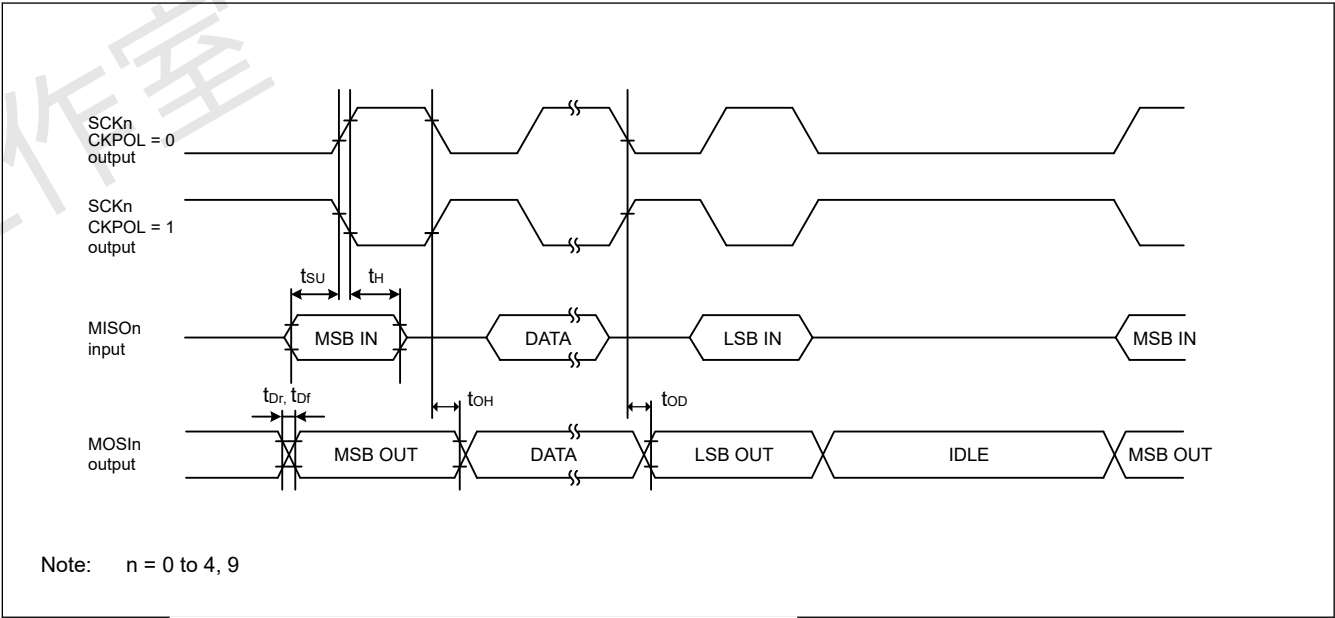
Figure 2.29 CKPH=1时主机的SCI简单SPI模式时序
