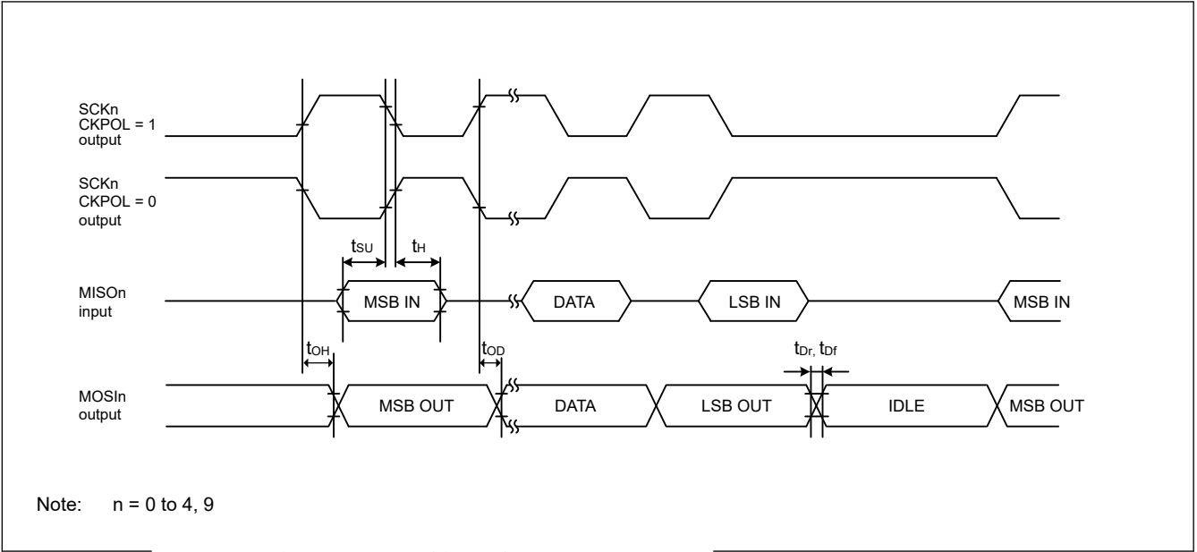
Figure 2.30 CKPH=0时主机的SCI简单SPI模式时序
