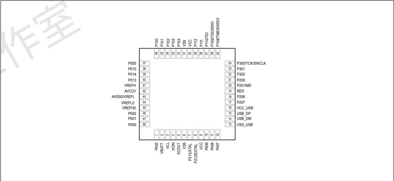
Figure 1.6 QFN48引脚的引脚分配
