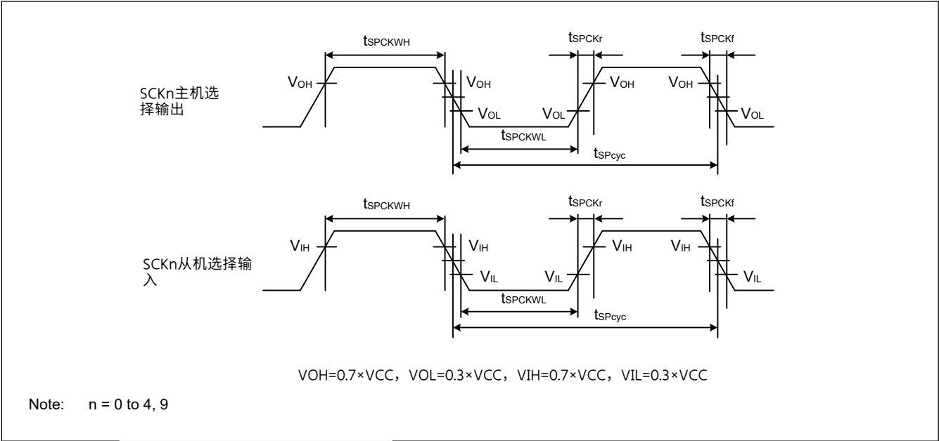
Figure 2.28 SCI简单SPI模式时钟时序
