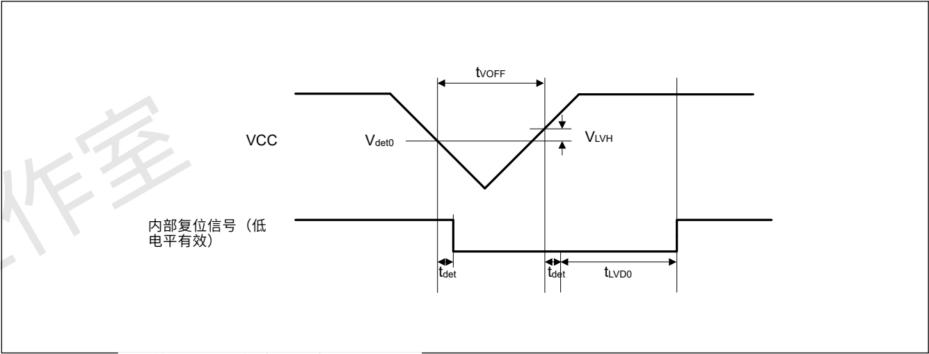
Figure 2.57 电压检测电路时序 (V det0 )
