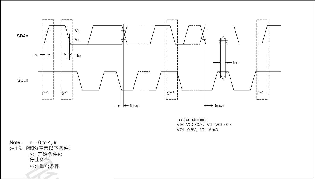
Figure 2.33 SCI简单IIC模式时序
