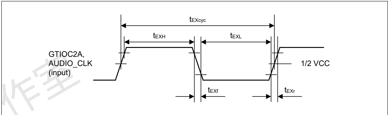
Figure 2.45 时钟输入时序
