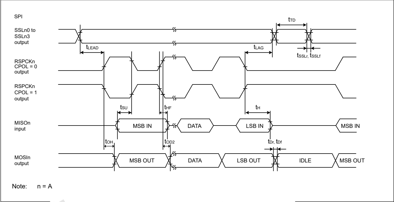
Figure 2.38 当CPHA=1且比特率设置为PCLKA2时，主机的RSPI时序
