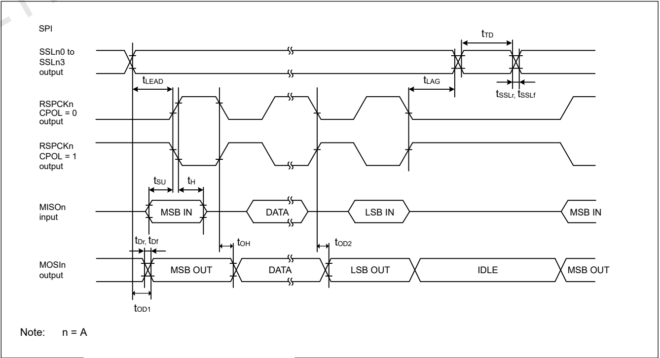
Figure 2.35 CPHA=0时主机的SPI时序
