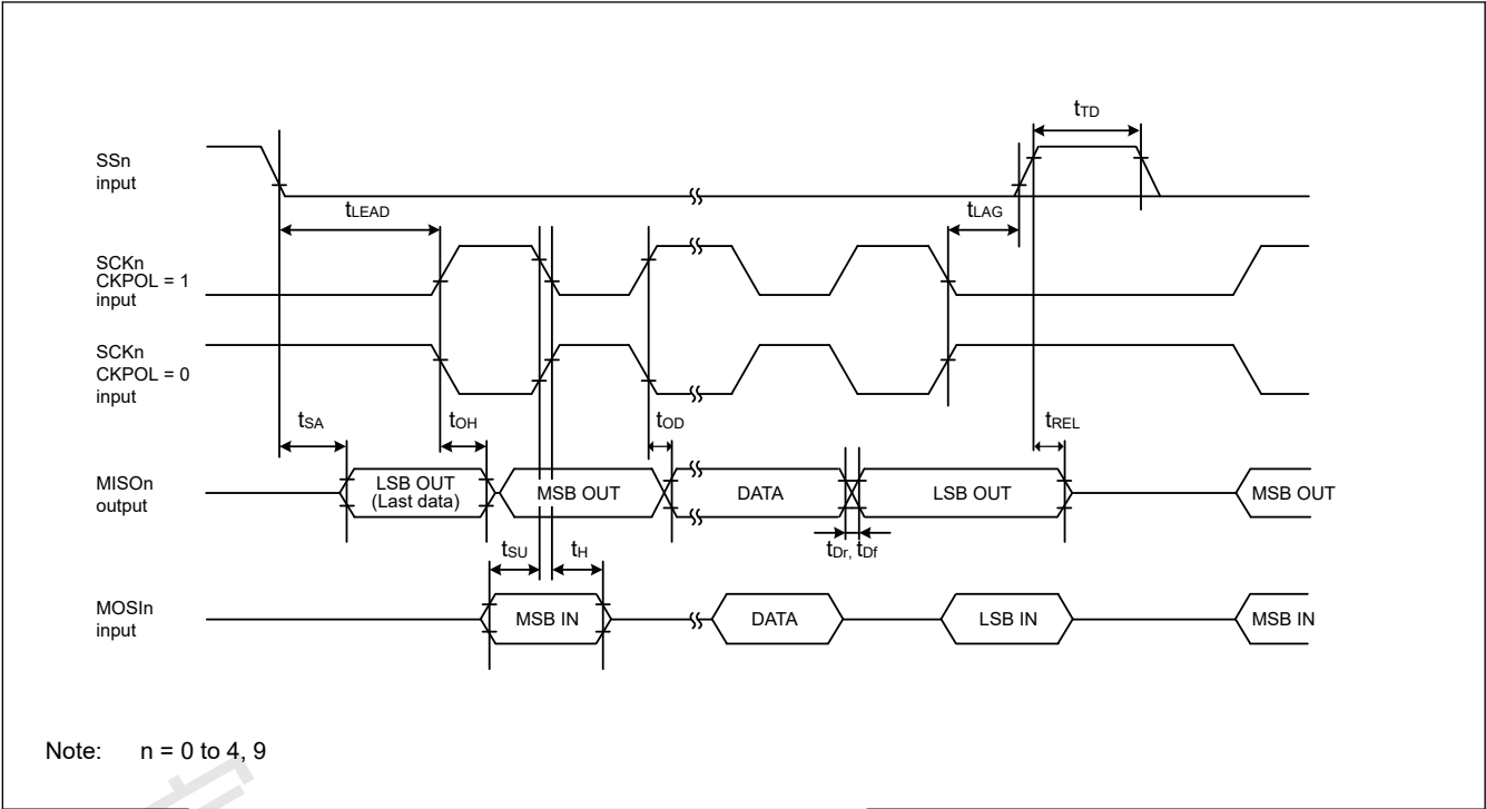
Figure 2.32 CKPH=0时从机的SCI简单SPI模式时序
