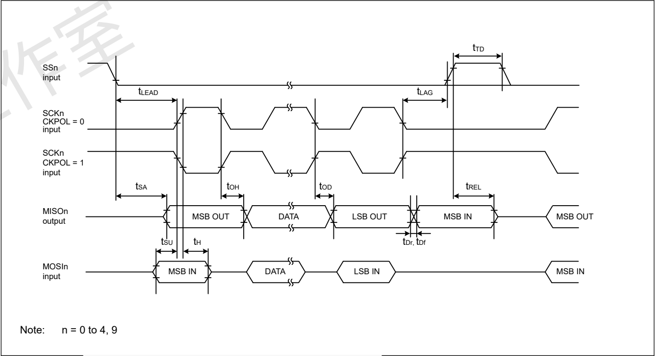
Figure 2.31 CKPH=1时从机的SCI简单SPI模式时序
