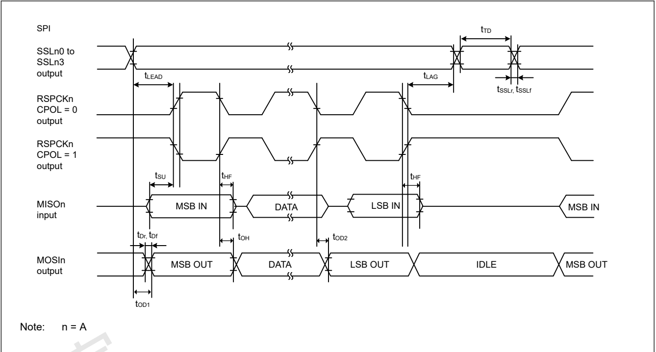
Figure 2.36 当CPHA=0且比特率设置为PCLKA/2时主设备的SPI时序
