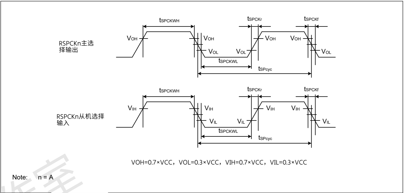
Figure 2.34 SPI时钟时序
