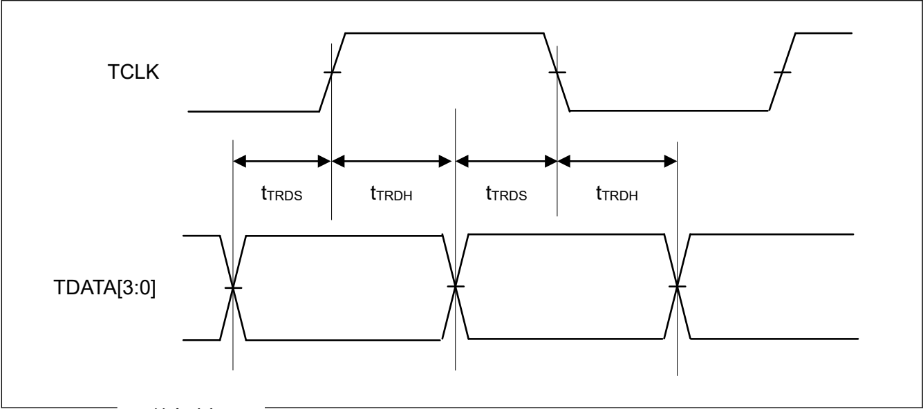
Figure 2.71 ETM输出时序
