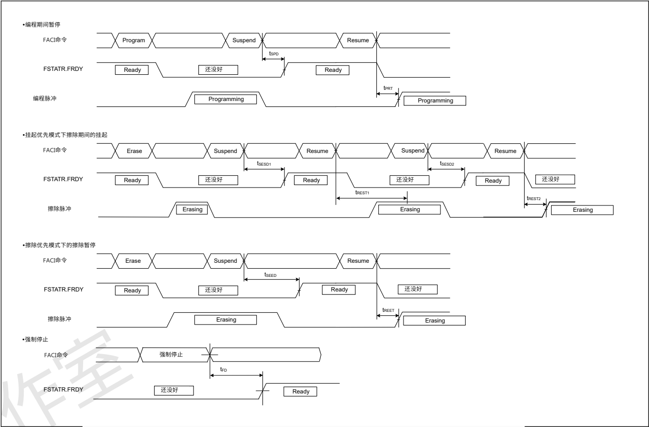
Figure 2.62 闪存编程和擦除的暂停和强制停止时序
