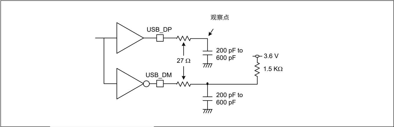
Figure 2.51 低速模式下的测试电路
