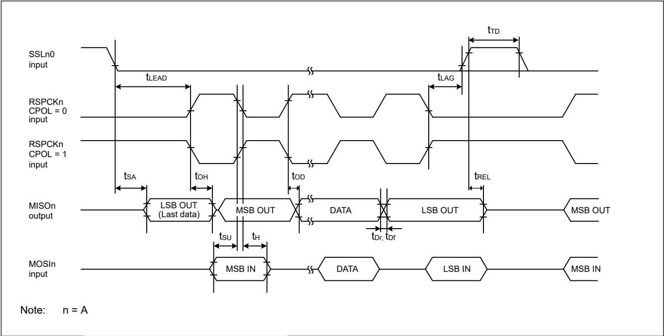
Figure 2.40 CPHA=1时从机的SPI时序
